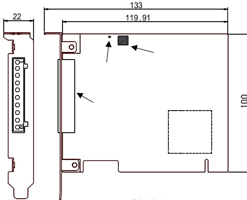
図 製品外形図
